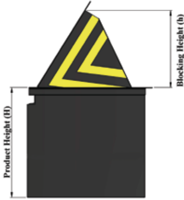
نموذج رؤية جانبية Model Side View
