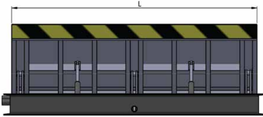
نموذج رؤية امامية Model Front View
