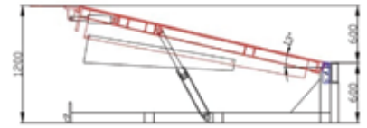
نموذج منصة تحميل مفتوحة Model Open View
