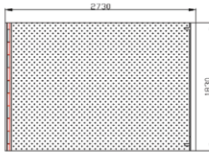
نموذج منصة تحميل من الأعلى Model Top View
