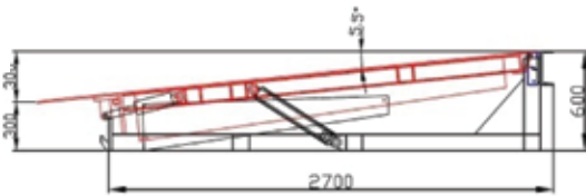
نموذج منصة تحميل مغلقة Model Close View
