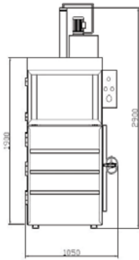
نموذج عرض من الأمام Model Front View
