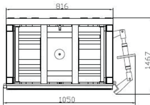
نموذج عرض من الاعلي Model Top View
