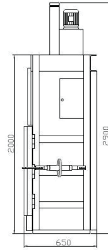
نموذج عرض من الجانب Model Side View
