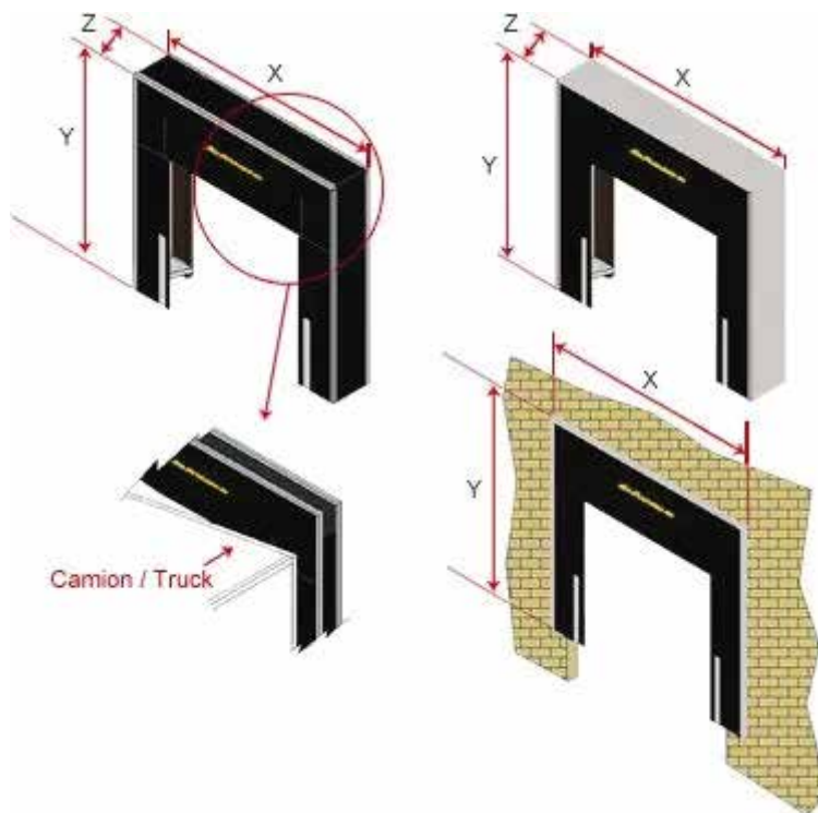
نموذج اغطية البوابات Model Dock shelter
