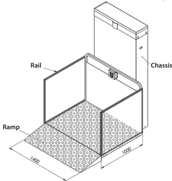
نموذج عرض من الأمام Model Front View
