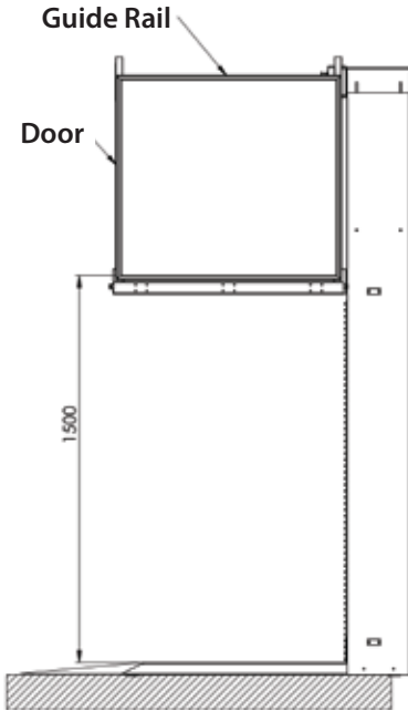
نموذج عرض من الجانب Model Side View
